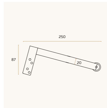
Door Selector
