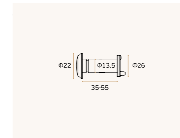
Door Viewer
